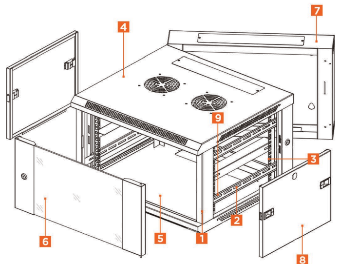
Οπίσθιο πλαίσιο περιστροφής επιτρέπει στο περίβλημα να απομακρύνεται από τον τοίχο
